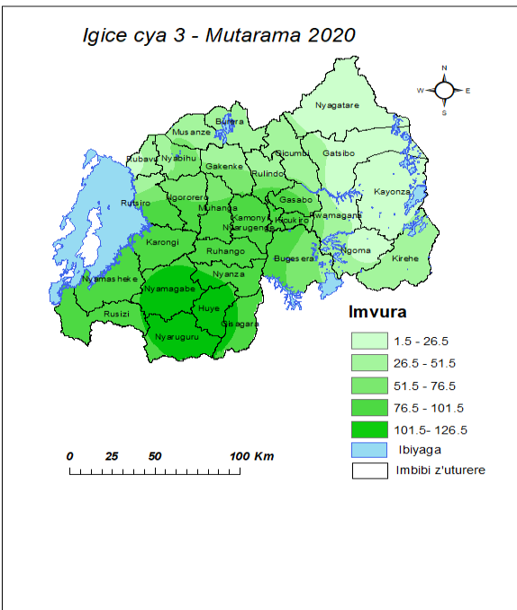
Ishusho1: Ingano y'Imvura muri mm
