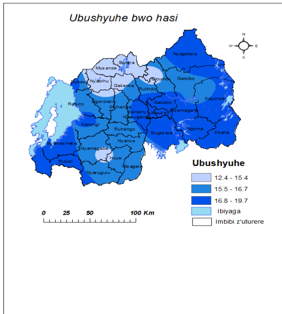
Ishusho ya 6: Ubushyuhe bwo hasi
