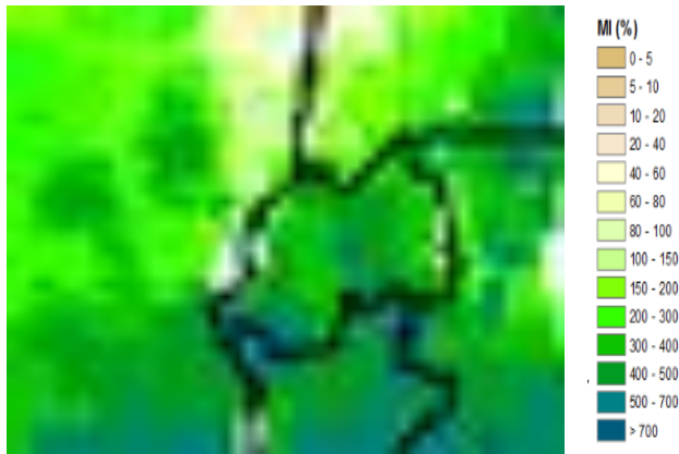
Ishusho 4: Ubuhehere bw'ubutaka
