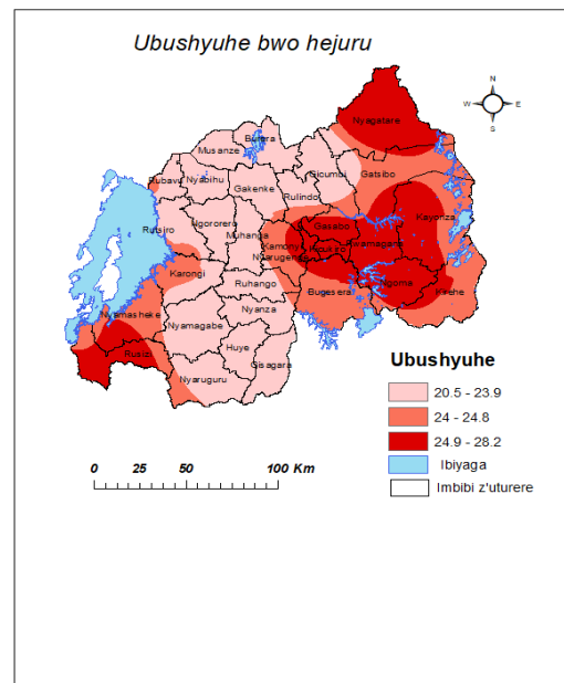
Ishusho ya 5: Ubushyuhe bwo hejuru
