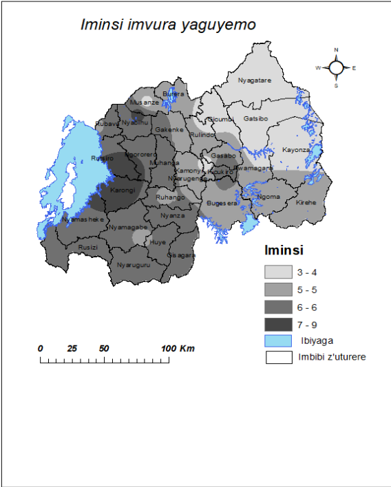
Ishusho 3: Umubare w'iminsi imvura yaguyemo
