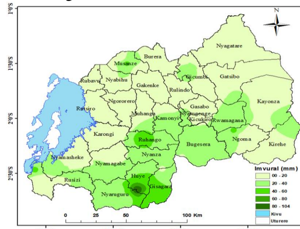
Ikarita ya 1: Ingano y'Imvura yaguye mu gice cya gatatu cya Gashyantare 2021
