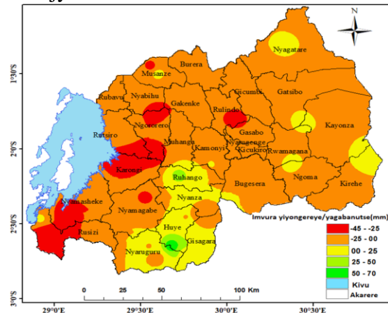
Ikarita 2 : Kwiyongera no kugabanuka kw'imvura mu gice cya gatatu cya Gashyantare 2021
