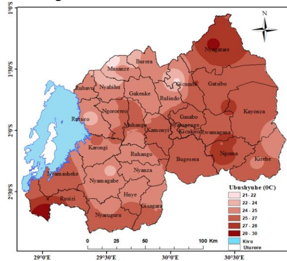
Ikarita ya 4: Ubushyuhe bwo hejuru
