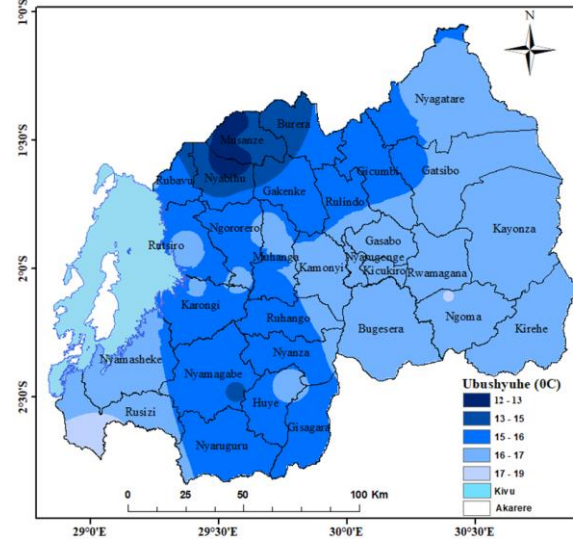
Ikarita ya 5: Ubushyuhe bwo hasi
