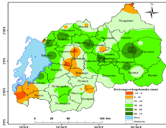
Ikarita 2: Kwiyongera no kugabanuka kwimvura mugice cya mbere cya Mutarama 2021
