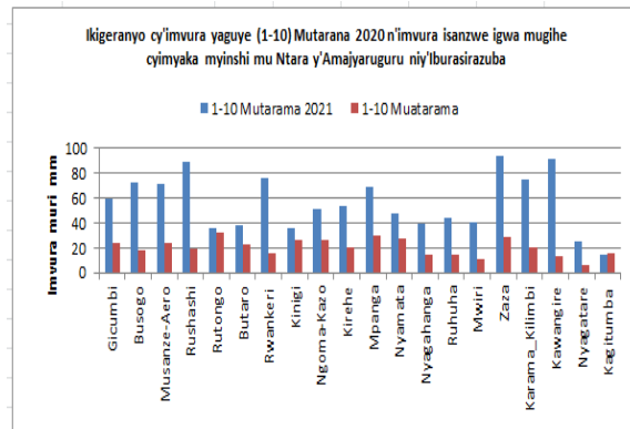
Ishusho 2: ikigereranyo cy'imvura mu ntara y'Amajyaruguru niy'Iburasirazuba
