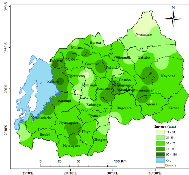
Ikarita ya 1: Ingano y'Imvura yaguye mu gice cya mbere cya Muatarama 2021
