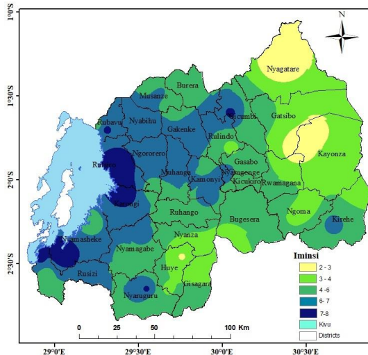
Ikarita ya 3: Umubare w'iminsi imvura yaguyemo
