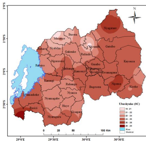
Ikarita ya 4: Ubushyuhe bwo hejuru
