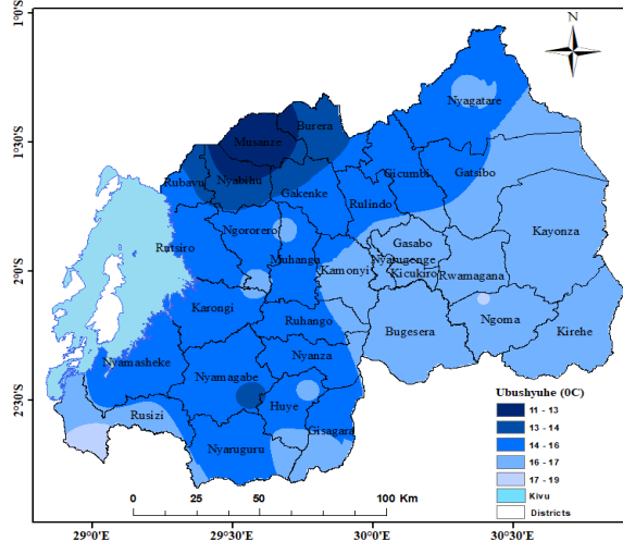
Ikarita ya 5: Ubushyuhe bwo hasi
