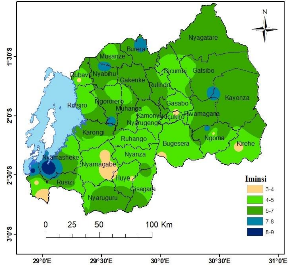
Ikarita ya 3: Umubare w'iminsi imvura yaguyemo
