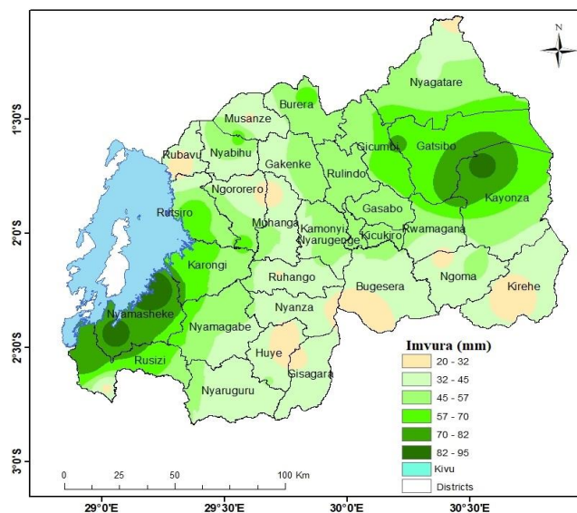
Ikarita ya 1: Ingano y'Imvura yaguye mu gice cya gatatu cy'Ugushyingo 2020
