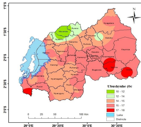
Ikarita ya 5: Ubushyuhe bwo hasi
