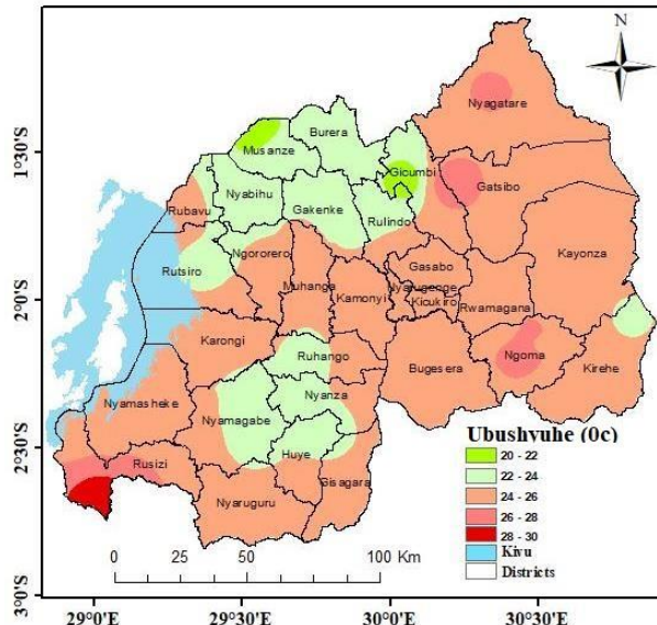
Ikarita ya 4: Ubushyuhe bwo hejuru
