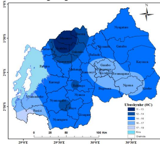
Ikarita ya 5: Ubushyuhe bwo hasi
