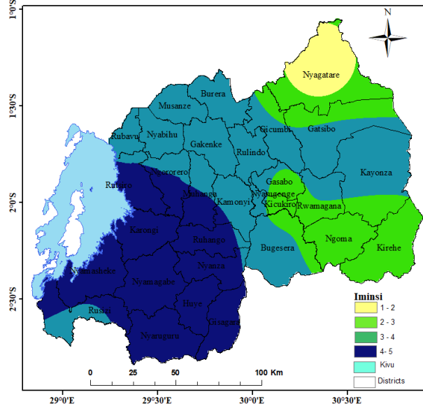
Ikarita ya 3: Umubare w'iminsi imvura yaguyemo
