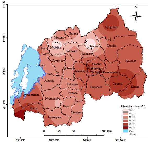
Ikarita ya 4: Ubushyuhe bwo hejuru
